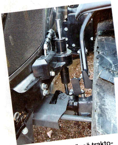
↑ Kuormauskäytössä traktorin vakautta lisää huomattavasti etuakselin keinun jäykistäminen. Kuvassa Jaken toteutustapa hydraulisynterillä.
